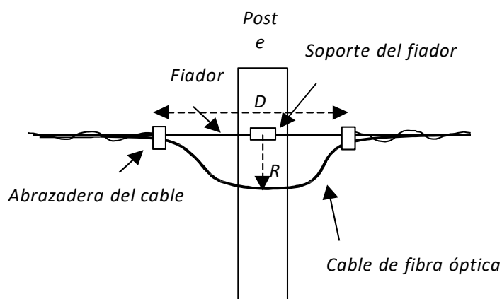
Figura 10 Fijación del cable.
