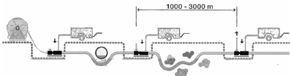
Figura: Tendido mediante Blowing
