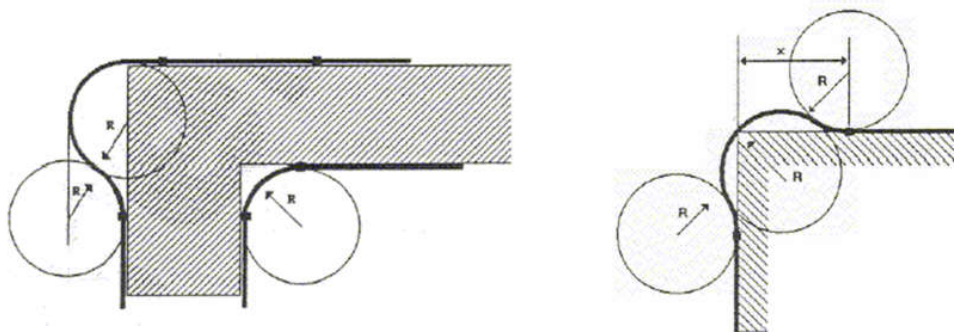
Figura: Criterios de curvatura para tendido en fachada (R = radio de curvatura del cable)
