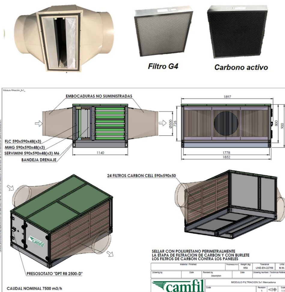
Unidad de Filtración marca CAMFIL modelo T3 PLUS 3010 REV-00
